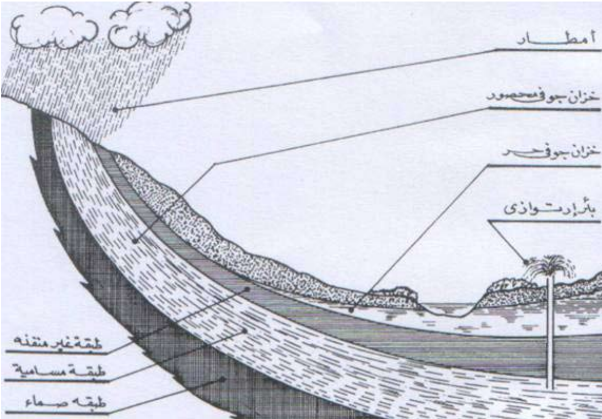
رسم توضيحي يبين طريقة تكون الخزان الجوفي بنوعيه الحر والمحصور
