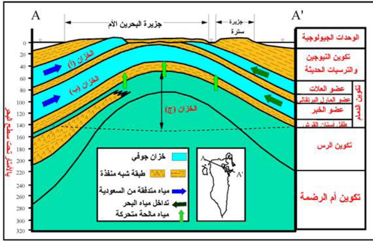
قطاع هيدروولوجي يبين توزيع الخزانات الجوفية في البحرين (زباري 1996م)
